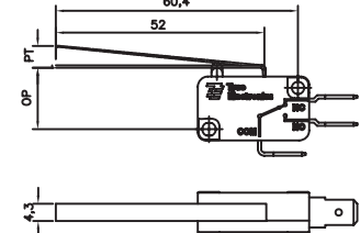
long lever
